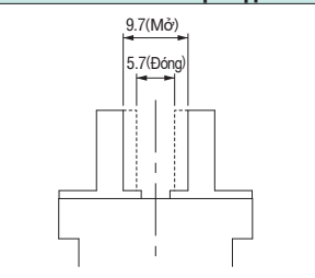
MHZ2-10SN (Loại hợp)
