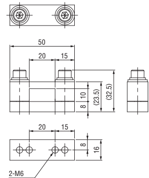
Slide bracket • 25-25
