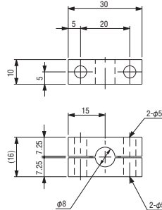
Bracket • W • φ8
