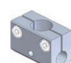
Khớp nối T #1 • \phi 8 \phi 12 Mã đặt hàng. 131105 MODEL N01861-303 ● Khối lượng : 22.6g
