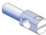
Khớp gá xoay • φ 12 • 12AL Mã đặt hàng. 131567 MODEL N01864-301L ● Khối lượng : 15.0g
