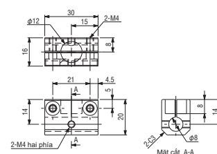
Khớp nối T #1 • \phi 8 \phi 12 Mã đặt hàng. 131105 MODEL N01861-303 ● Khối lượng : 22.6g
