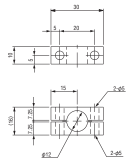
Khớp gá • W • \phi 12
