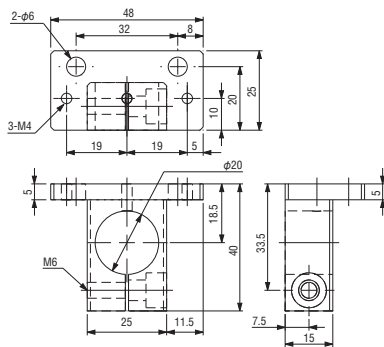
Khớp gá • \phi 20
