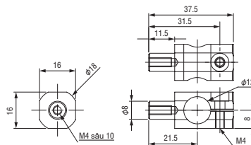
Khớp gá xoay • φ 12 • 8 A Mã đặt hàng. 131169 MODEL N01864-302 ● Khối lượng : 11.9g
