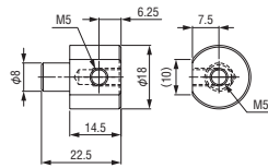
Khớp gá xoay • φ 8 • M5A Mã đặt hàng. 131164 MODEL N01864-202 ● Khối lượng : 10.0g
