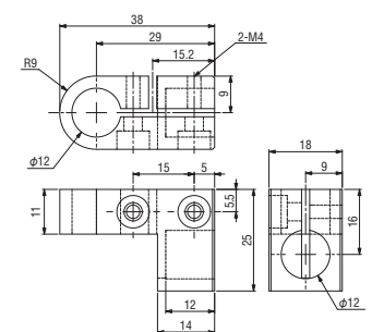
Khớp gá xoay • φ 12 • 12B Mã đặt hàng. 131605 MODEL N01864-102A ● Khối lượng : 22.0g
