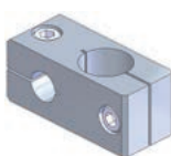
Khớp chéo • \phi 20 \phi 12 Mã đặt hàng. 131100 MODEL N01861-204 ● Khối lượng : 72.0g
