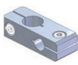
Khớp chéo • \phi 12 \phi 8 Mã đặt hàng. 131098 MODEL N01861-201 ● Khối lượng : 16.8g
