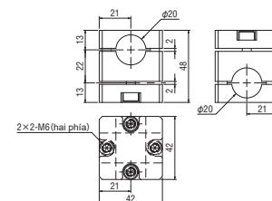
Khớp chéo • \phi 20 \phi 20 (lắp sau) Mã đặt hàng. 131570 MODEL N01861-206A ● Khối lượng : 160.0g
