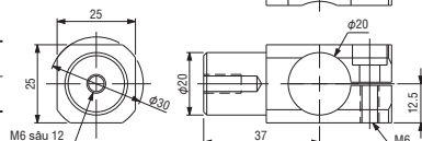
Khớp gá xoay • φ 20 • 20A Mã đặt hàng. 131171 MODEL N01864-304 ● Khối lượng : 50.7g
