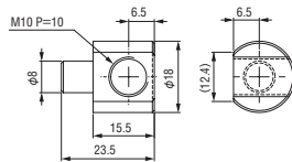
Khớp gá xoay • φ 12 • 8 A Mã đặt hàng. 131169 MODEL N01864-302 ● Khối lượng : 11.9g
