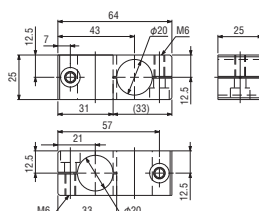
Khớp chéo • \phi 20 \phi 20 Mã đặt hàng. 131101 MODEL N01861-206 ● Khối lượng : 50.3g
