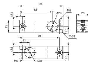
Khớp chéo • dài • \phi 20 \phi 20 Mã đặt hàng. 131573 MODEL N01861-206B ● Khối lượng : 109.0g
