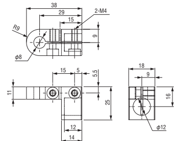
Khớp gá xoay • φ 12 • 12B Mã đặt hàng. 131605 MODEL N01864-102A ● Khối lượng : 22.0g
