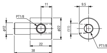
Khớp gá xoay • φ 12 • PT1/8A Mã đặt hàng. 131166 MODEL N01864-204 ● Khối lượng : 24.6g
