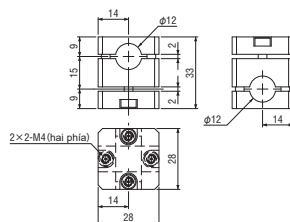
Khớp chéo • \phi 12 \phi 12 (lắp sau) Mã đặt hàng. 131569 MODEL N01861-202A ● Khối lượng : 51.3g
