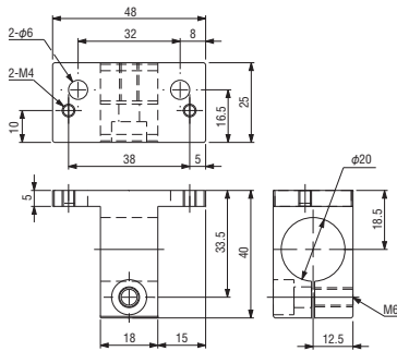
Khớp gá • TV • \phi 20 • cho MCD
