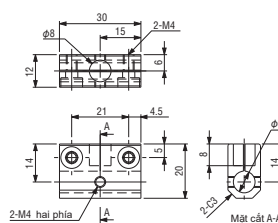
Khớp nối T #1 • \phi 8 \phi 8 Mã đặt hàng. 131108 MODEL N01861-306 ● Khối lượng : 12.5g
