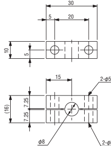
Khớp gá • W • \phi 8
