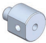
Khớp gá xoay • φ 8 • M5A Mã đặt hàng. 131164 MODEL N01864-202 ● Khối lượng : 10.0g
