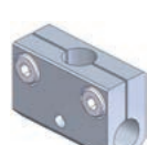
Khớp nối T #1 • \phi 8 \phi 8 Mã đặt hàng. 131108 MODEL N01861-306 ● Khối lượng : 12.5g
