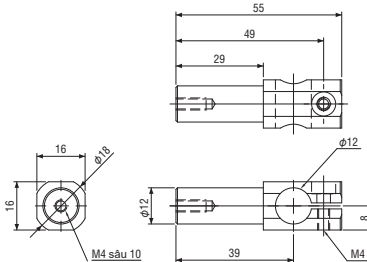
Khớp gá xoay • φ 12 • 12AL Mã đặt hàng. 131567 MODEL N01864-301L ● Khối lượng : 15.0g
