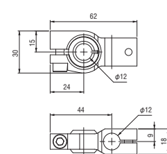
Khớp chéo cầu \phi 12 Mã đặt hàng. 054346 MODEL F-CROSS-12 ● Khối lượng : 45.0g
