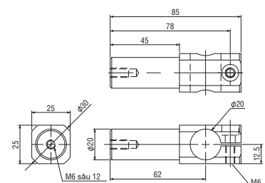
Khớp gá xoay • φ 20 • 20AL Mã đặt hàng. 131568 MODEL N01864-304L ● Khối lượng : 80.0g
