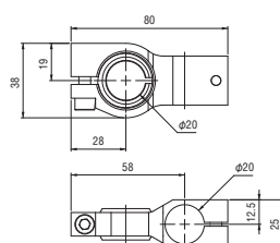
Khớp chéo cầu \phi 20 Mã đặt hàng. 054347 MODEL F-CROSS-20 ● Khối lượng : 72.0g
