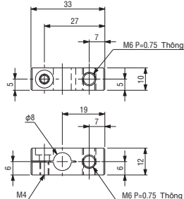
Khớp gá giác hút • φ 12 • PT1/8
