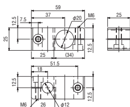
Khớp chéo • \phi 20 \phi 12 Mã đặt hàng. 131100 MODEL N01861-204 ● Khối lượng : 72.0g
