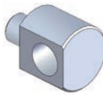
Khớp gá xoay • φ 8 • M10A Mã đặt hàng. 131435 MODEL N01864-201 ● Khối lượng : 8.0g
