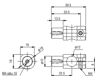
Khớp gá xoay • φ 12 • 12A Mã đặt hàng. 131168 MODEL N01864-301 ● Khối lượng : 14.6g
