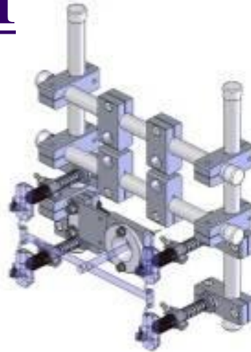
BẢN VẼ THIẾT KẾ
